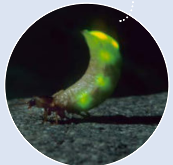
Glühwürmchen ( Lampyrisa splendida )
